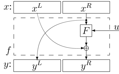
Σχήμα 5.3: Ένας γύρος Feistel πάνω από τη συνάρτηση F .
