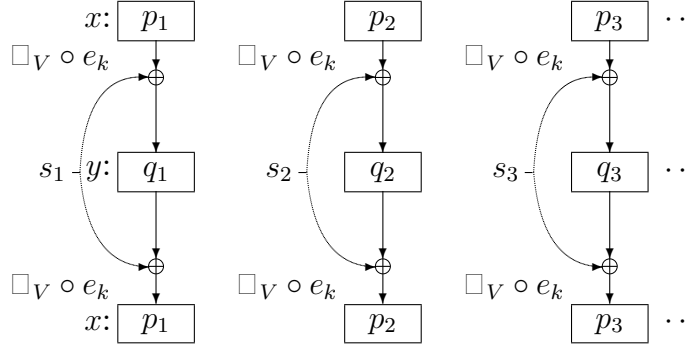
Σχήμα 5.13: Χρήση του DES με ανάδραση.
