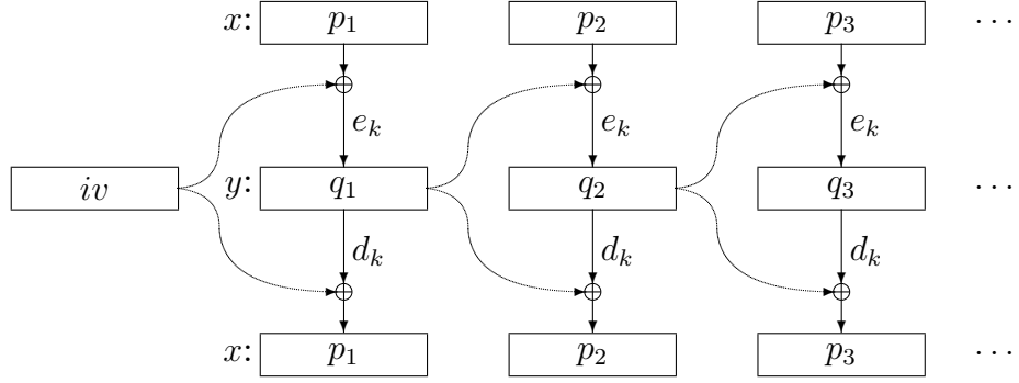
Σχήμα 5.12: Χρήση του DES με αλυσωτή σύνδεση των πακέτων. Το ένα από τα δύο κομμάτια δείχνει την κρυπτογράφηση (πάνω) και το άλλο την αποκρυπτογράφηση (κάτω).
