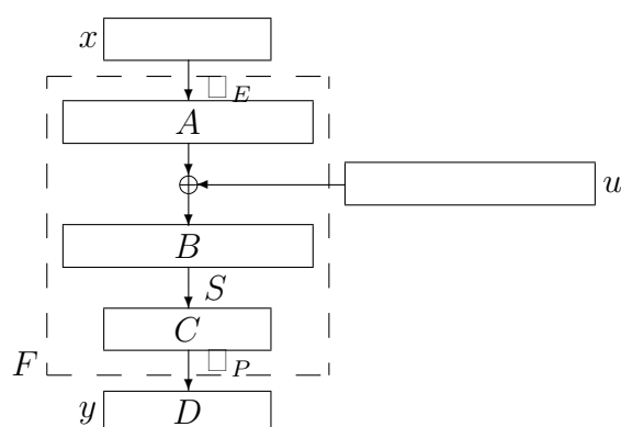
Σχήμα 5.7: Η συνάρτηση F πάνω από την οποία ορίζεται το Feistel δίκτυο \mathcal{F} του DES.
