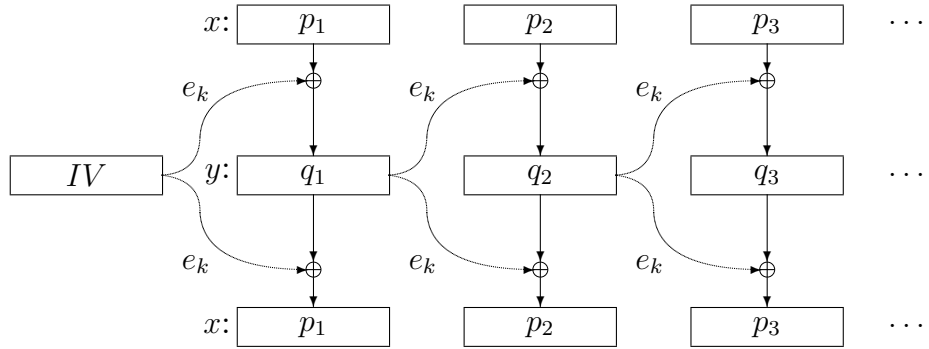
Σχήμα 5.17: Η λειτουργία με ανάδραση από τα κρυπτοκείμενα, όταν l = 64 .
