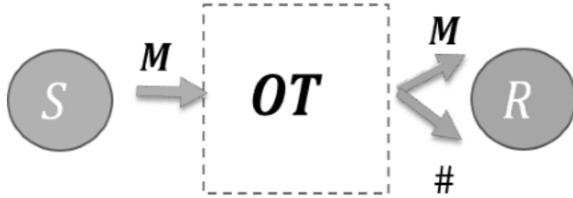
Σχήμα 9.2: Μη-Συνειδητή Μεταφορά
