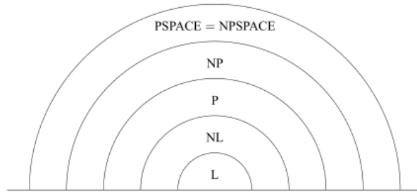
Σχήμα 3.1: Κλάσεις Πολυπλοκότητας
