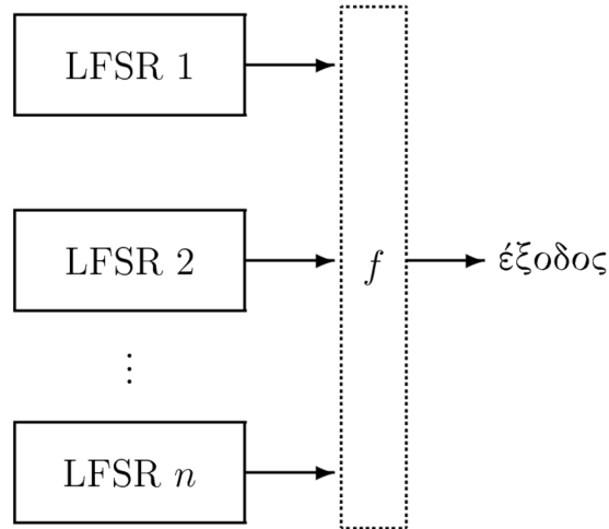
Σχήμα 5.31: Εφαρμογή μη γραμμικού συνδυαστή σε πολλούς LFSRs
