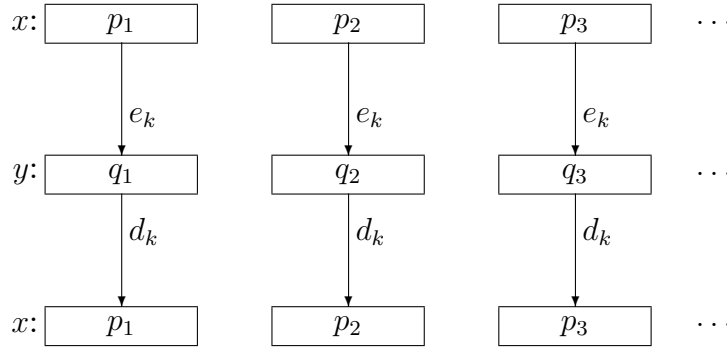
Σχήμα 5.11: Χρήση του DES ως ηλεκτρονικού βιβλίου κωδικών. Το ένα από τα δύο κομμάτια δείχνει την κρυπτογράφηση (πάνω) και το άλλο την αποκρυπτογράφηση (κάτω).
