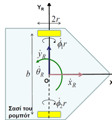
Διαφορικά οδηγούμενο ρομπότ.
