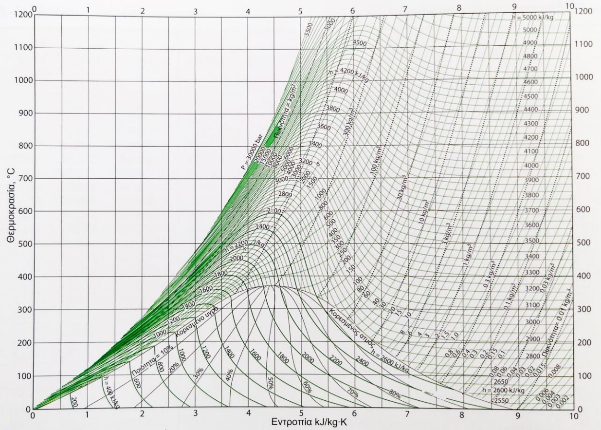
ΣΧΗΜΑ Α-9: Διάγραμμα T-s του νερού
