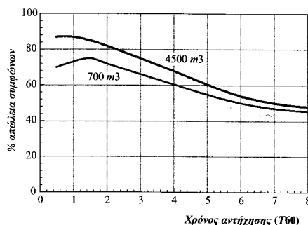
Σχήμα 7.3.10 Σχέση AL και T_{60} .
