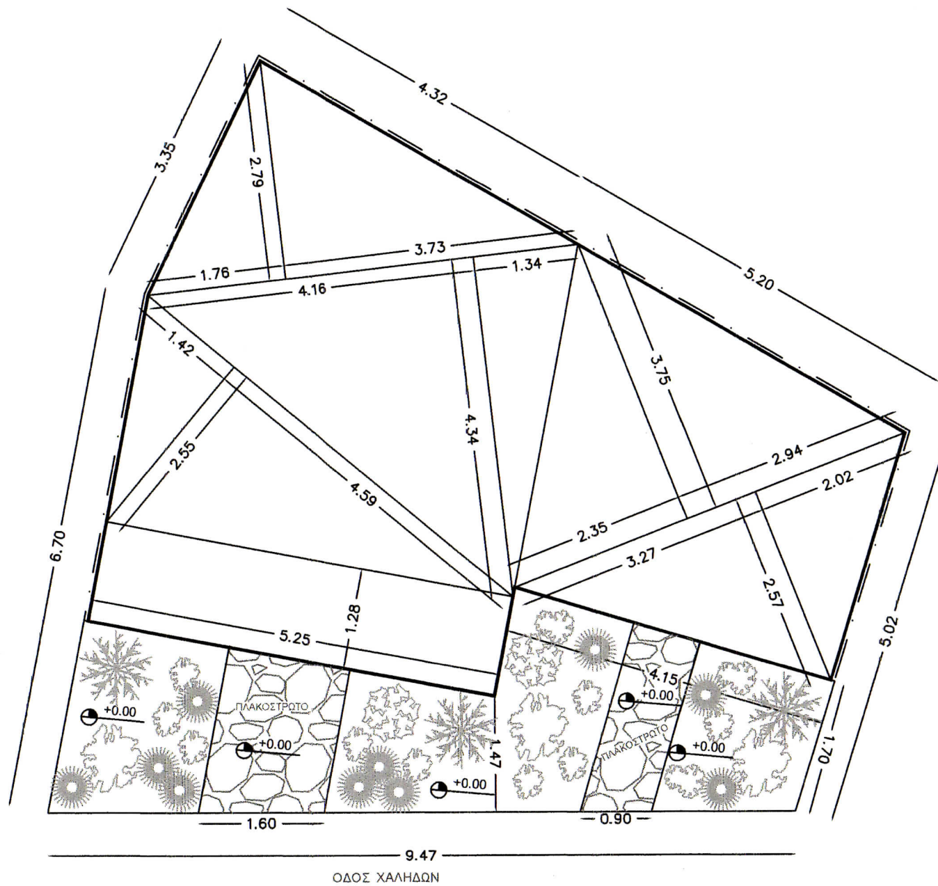
ΔΙΑΓΡΑΜΜΑ ΚΑΛΥΨΗΣ ΙΣΟΓΕΙΟΥ - ΔΙΑΜΟΡΦΩΣΗ ΑΚΑΛΥΠΤΟΥ ΧΩΡΟΥ
