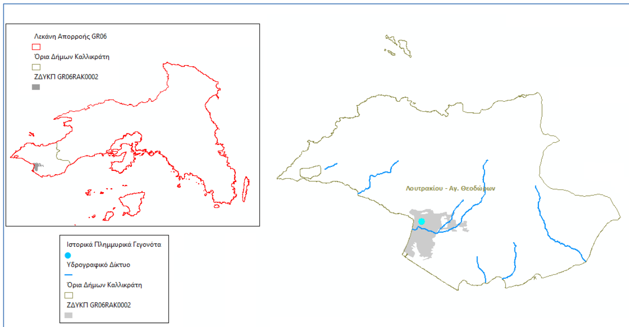
Σχήμα 7.11: Οικισμοί εντός ΖΔΥΚΠ GR06RAK0002 που επλήγησαν από τις πλημμύρες 21/10/1994
