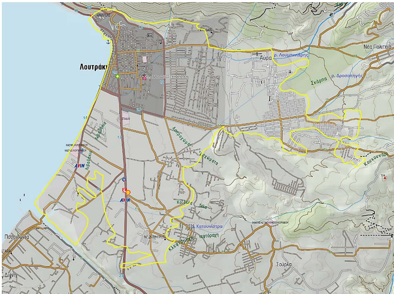
Σχήμα 7.9: Υδατορεύματα στην ΖΔΥΚΠ χαμηλή ζώνη Λουτρακίου
