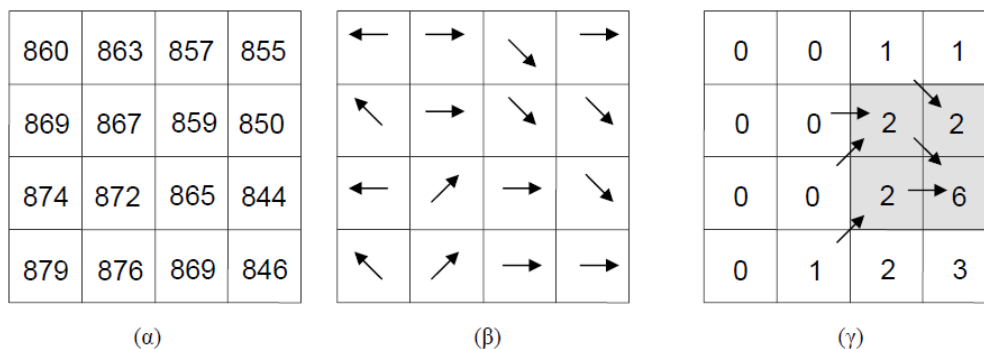
Σχήμα 5.11: Διαμόρφωση καννάβου συγκέντρωσης ροής
