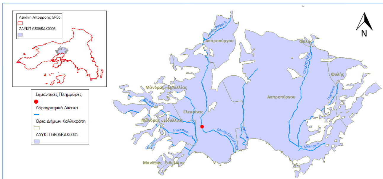
Σχήμα 7.28: Οικισμοί εντός ΖΔΥΚΠ GR06RAK0005 που επλήγησαν από τις πλημμύρες 01/01/1996.
