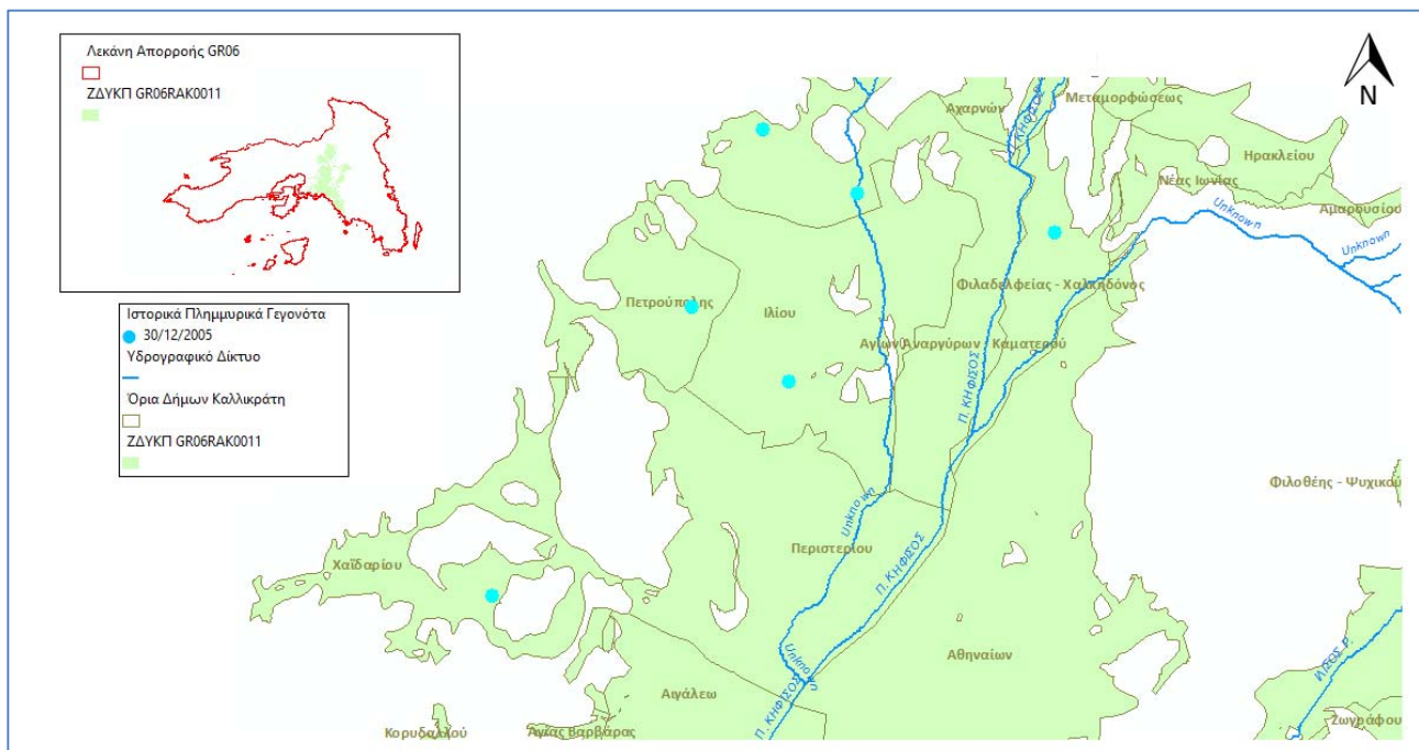
Σχήμα 7.55: Οικισμοί εντός ΖΔΥΚΠ GR06RAK0011 που επλήγησαν από τις πλημμύρες 30/12/2005
