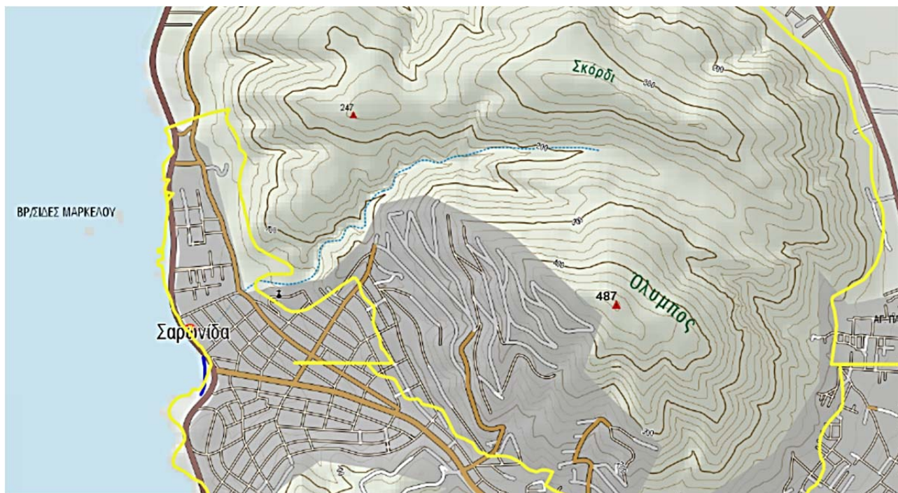
Σχήμα 7.6: Υδατόρευμα στην περιοχή Σαρωνίδας
