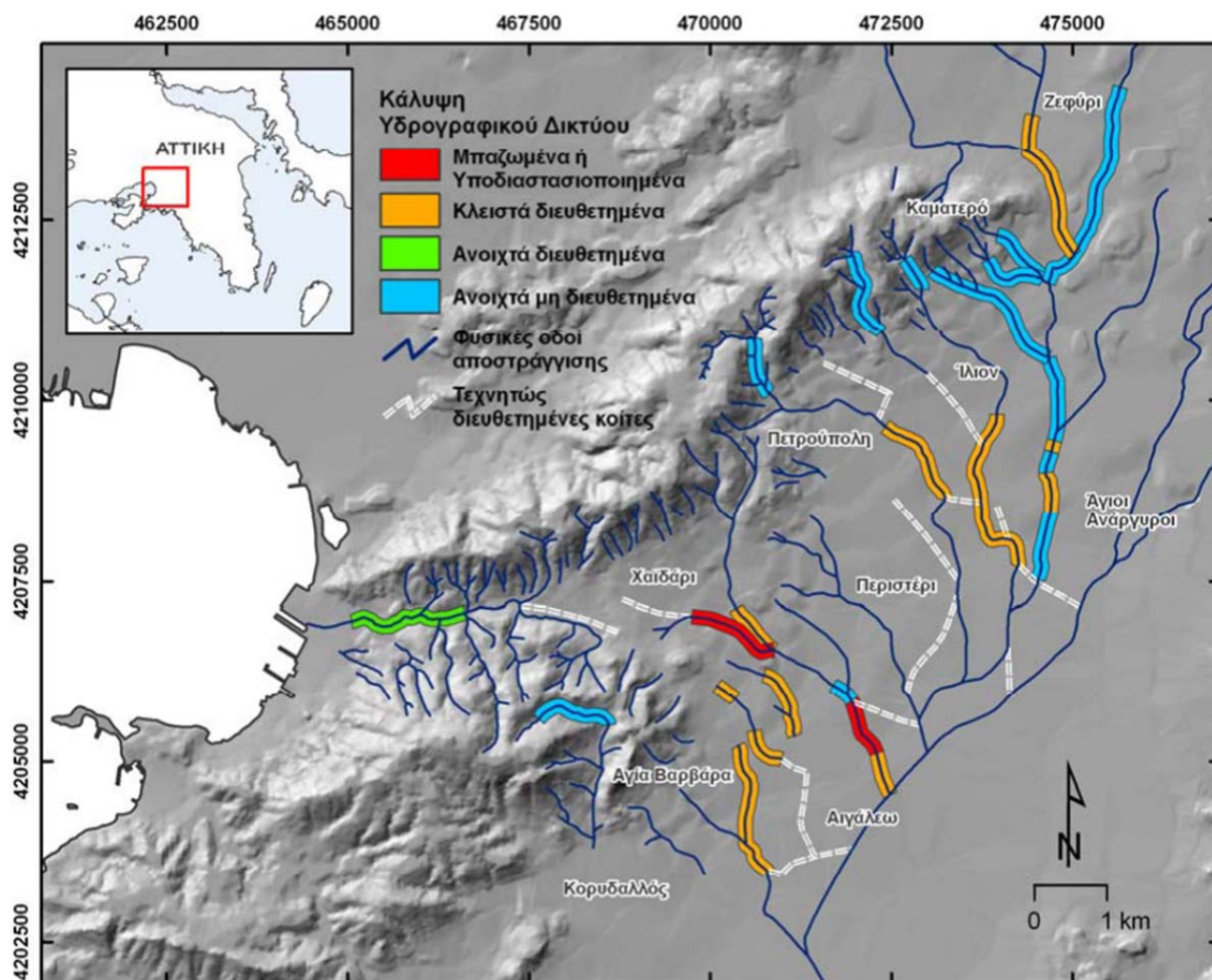
Σχήμα 7.64: Υδρογραφικό δίκτυο Δυτικής Αθήνας
