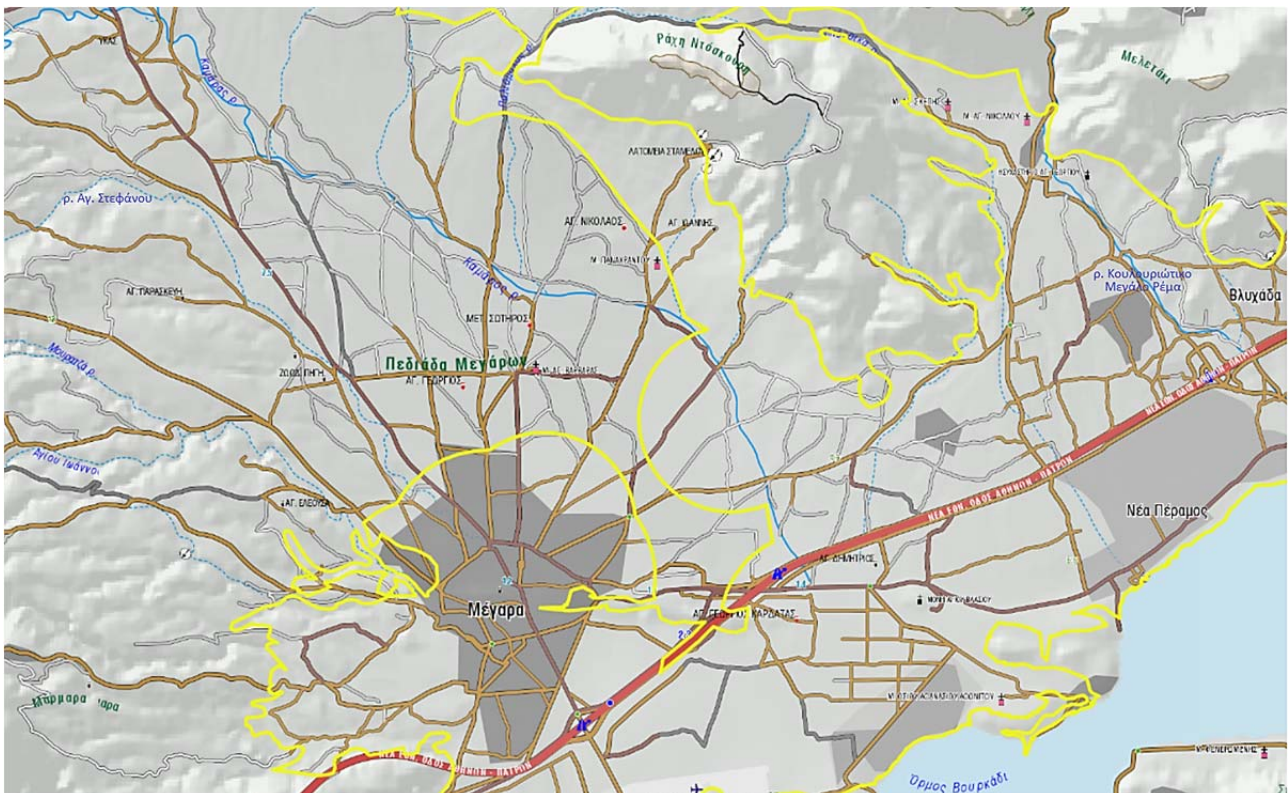
Σχήμα 7.23: Υδατορεύματα στην ΖΔΥΚΠ χαμηλή ζώνη Μεγάρων-Ν. Περάμου
