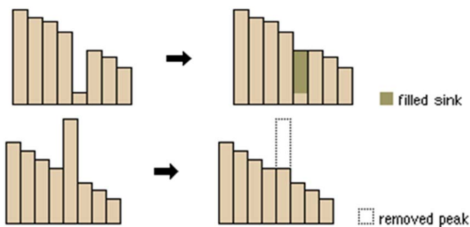
Σχήμα 5.4: Διόρθωση ατελειών του Ψηφιακού Μοντέλου Εδάφους
