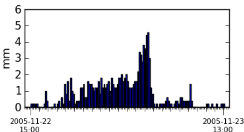
Σχήμα 7.36: 10λεπτη κατανομή της βροχόπτωσης στο σταθμό Πεντέλη
