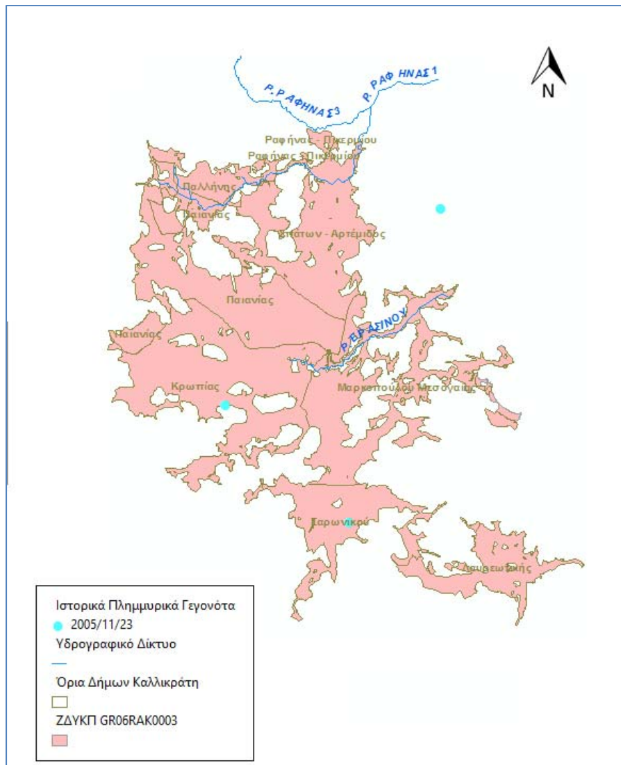
Σχήμα 7.17: Οικισμοί εντός ΖΔΥΚΠ GR06RAK0003 που επλήγησαν από τις πλημμύρες 23-24/11/2005.
