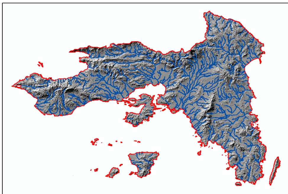
Σχήμα 5.12: Παραγόμενο επίπεδο συσσώρευσης ροής ΥΔ Αττικής
