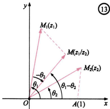
Τα τρίγωνα OAM_2 και OMM_1 είναι όμοια
