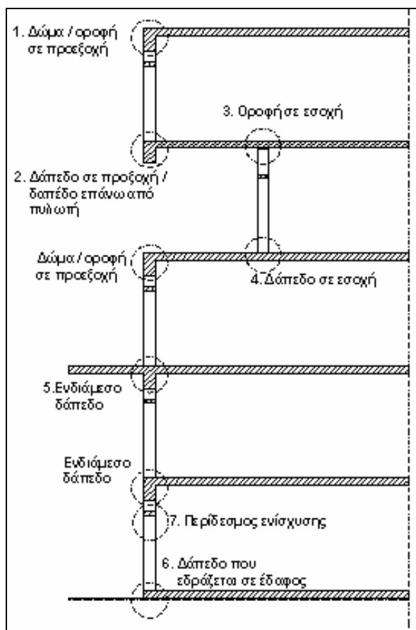
Σχήμα 6.2. Ενδεικτικές θέσεις εμφάνισης οριζόντιων θερμογεφυρών.
