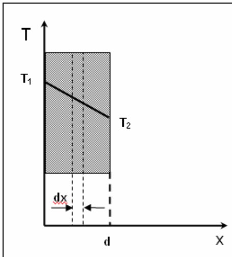
Σχήμα 2.2. Μεταφορά θερμότητας σε ομογενές επίπεδο υλικό.
